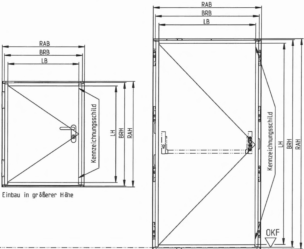
Ansicht Schließseite
